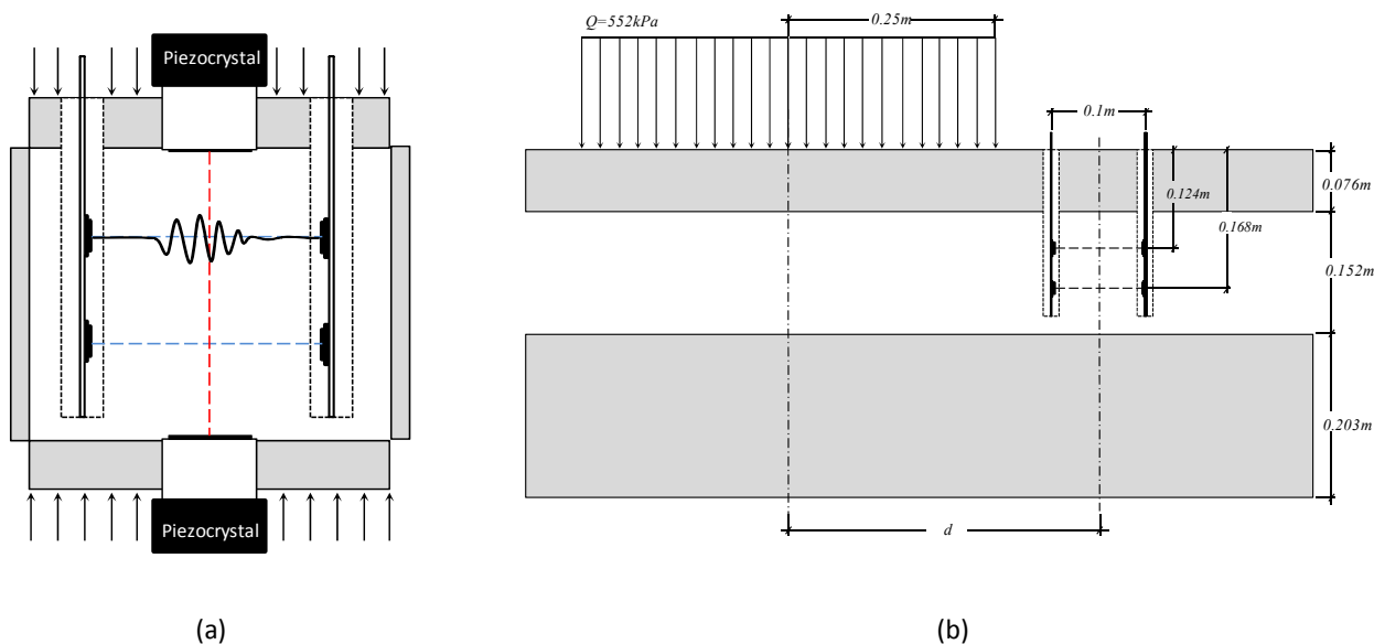
Figura 1: Sensores desarrollados para la determinación de la rigidez de bases granulares en función del estado de esfuerzos. El nuevo ensayo hace posible la medición directa del módulo de onda-P en (a) el laboratorio y (b) in-situ.
