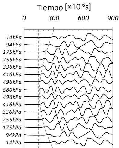
Figura 2: Evolución típica de las señales en función del estado de esfuerzos.
