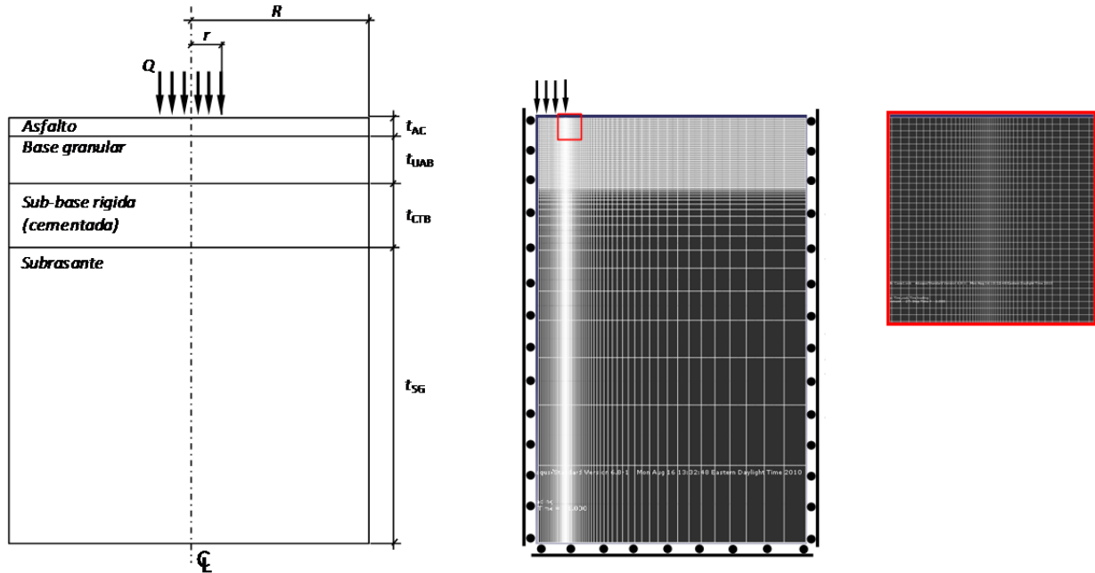
Figura 4: Geometría del pavimento flexible con rigidez invertida y modelos constitutivos usados para cada material.
